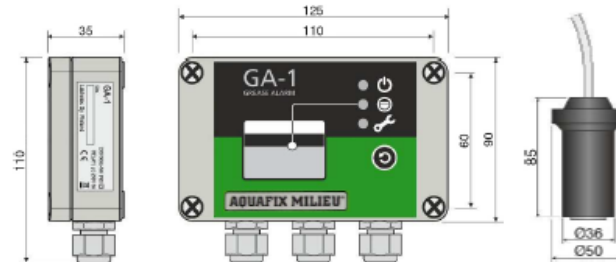
Afbeelding 7. Reguleenheid GA-1
