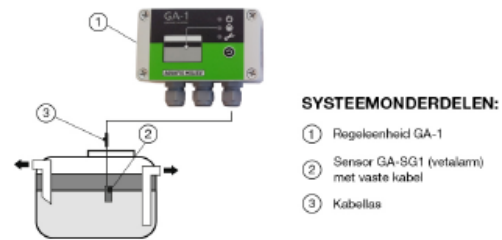
Afbeelding 1. Bewaking vetafscheider met alarmtoestel GA-1
